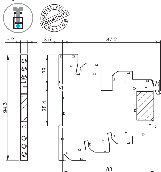
Typ 39.40 39.41 Käfigklemmen
