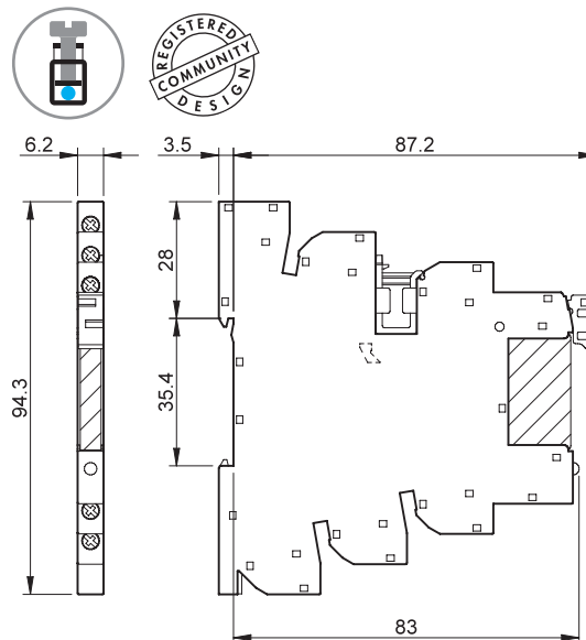
Typ 39.30/39.30.3 39.31/39.31.3 Käfigklemmen
