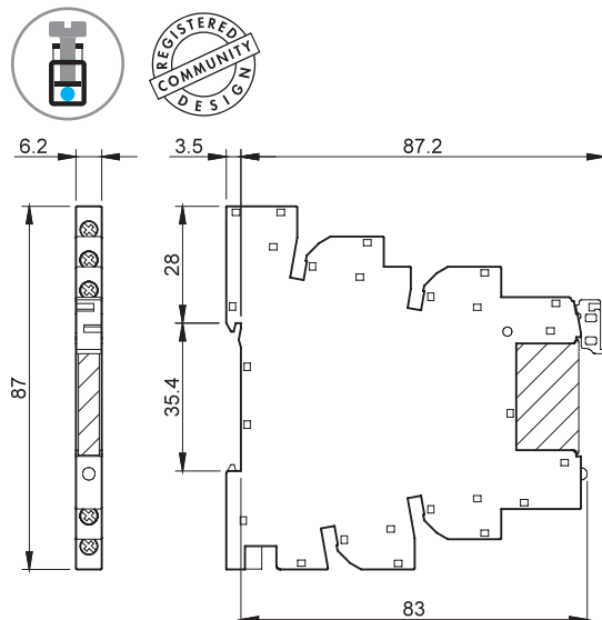
Typ 39.10/39.20 39.11/39.21 Käfigklemmen
