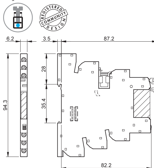
Typ 39.80 39.81 Käfigklemmen
