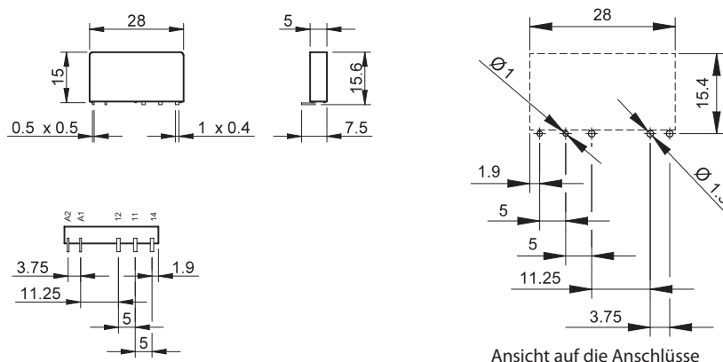
Ansicht auf die Anschlüsse
