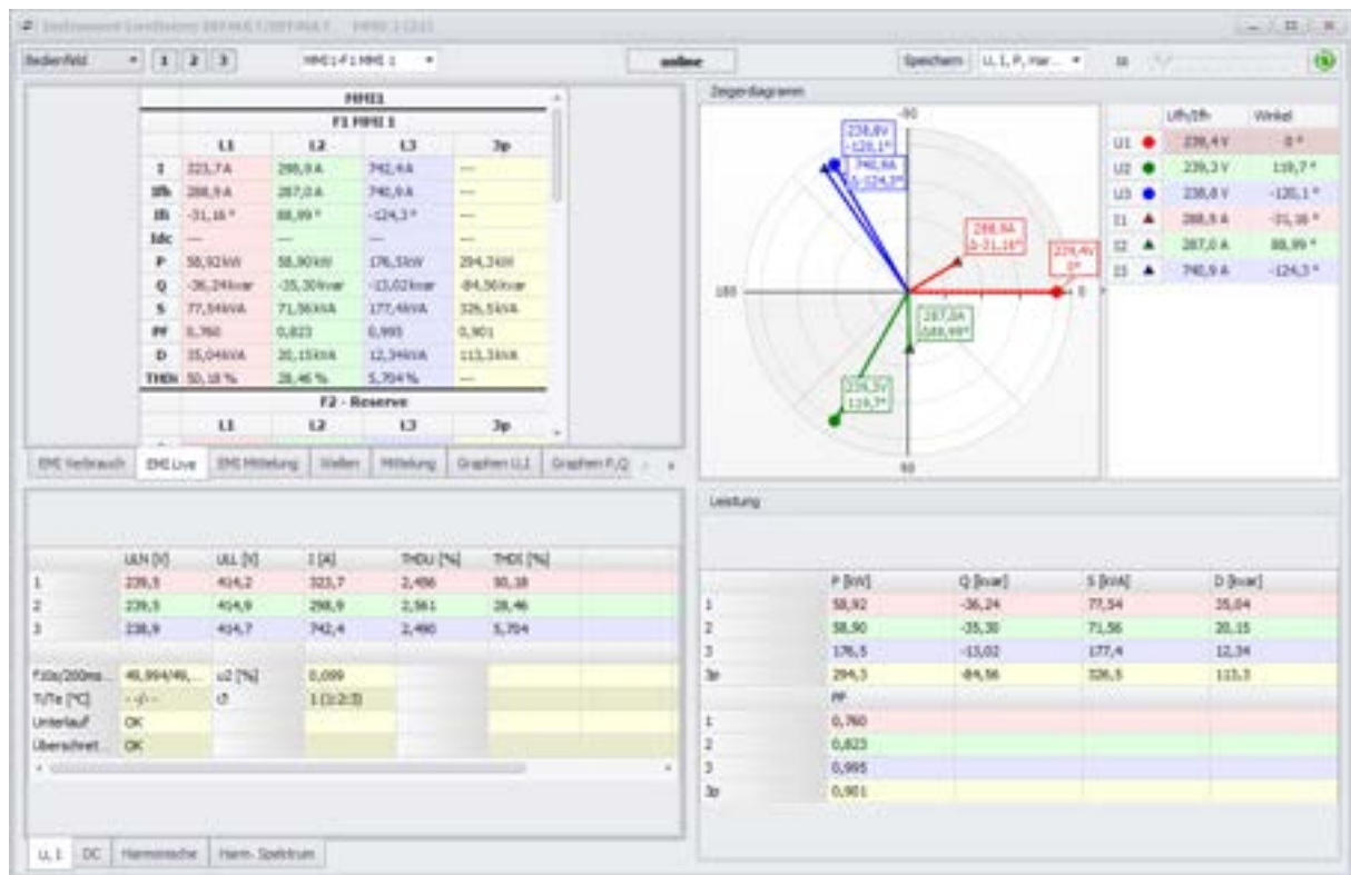
Abbildung 4: ENVIS.Daq – LiveDaten-Fenster
