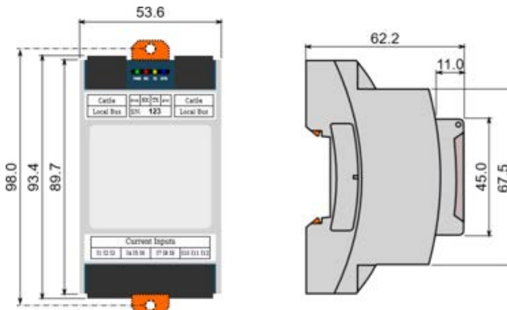
Abbildung 1: Abmessungen MMI12
