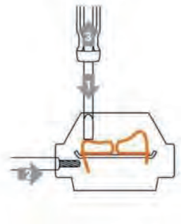
Schraubenlose Anschlusstechnik dank Federzugklemme „Cage Clamp“ ® (Front oder Top)
