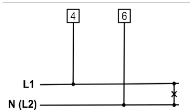
Direktschaltung
