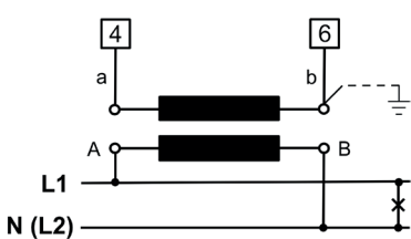
Wandlerschaltung
