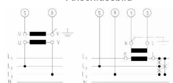
Anschlussbild
