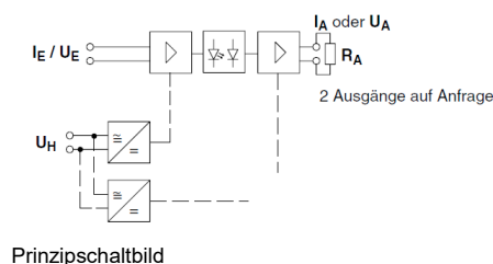
Prinzipschaltbild
