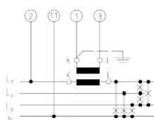
Klemmenbelegung
