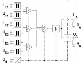
Prinzipialschaltbild (Beispiel)
