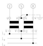
Anschlussbild
