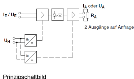
Prinzipialschaltbild
