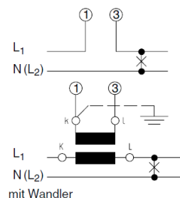
Anschlussbild
