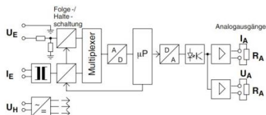
Prinzipialschaltbild (Beispiel)
