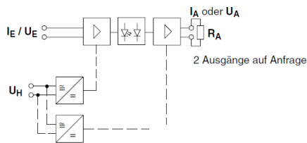
Prinzipschaltbild
