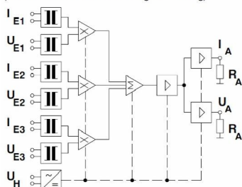
Principalschaltbild (Beispiel)
