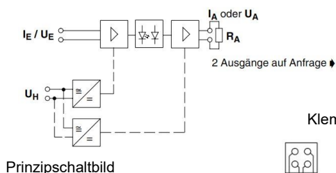
Prinzipialschaltbild
