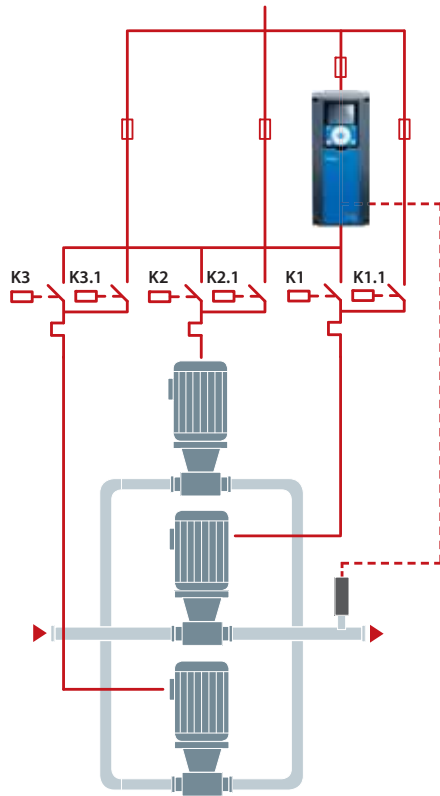
Einzeltriebssystem
