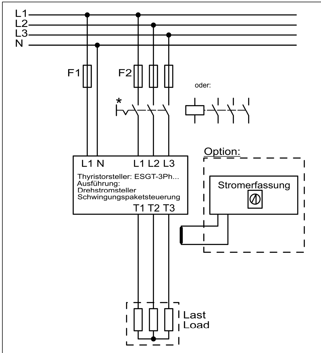
Abbildung 3: Grundschaltung
