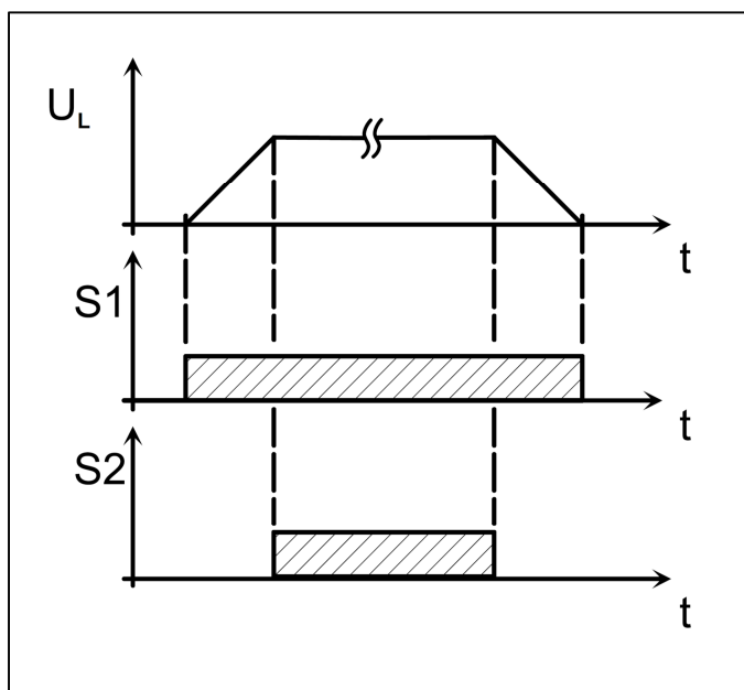
Abbildung 5: Zusammenhang U_L , S1 und S2
