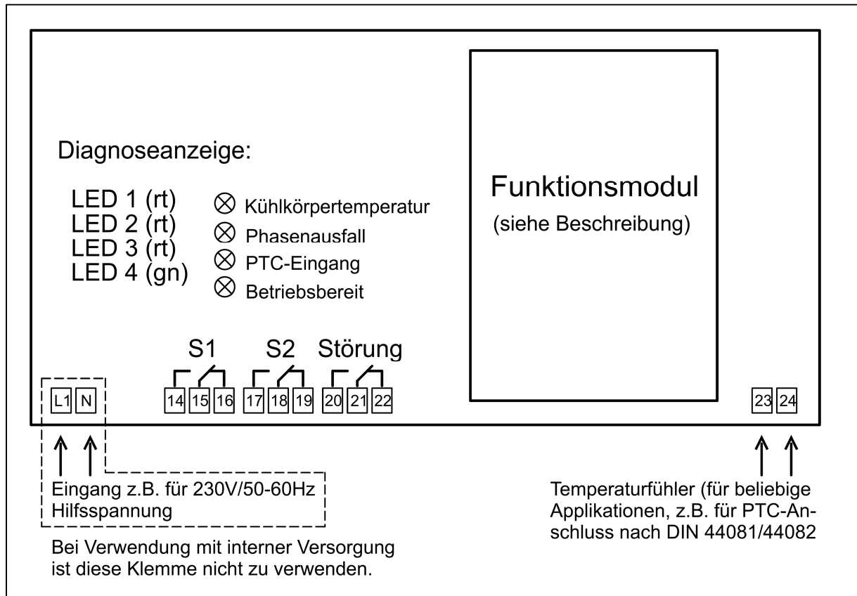
Abbildung 4: Prinzipieller Aufbau der Steuerplatine
