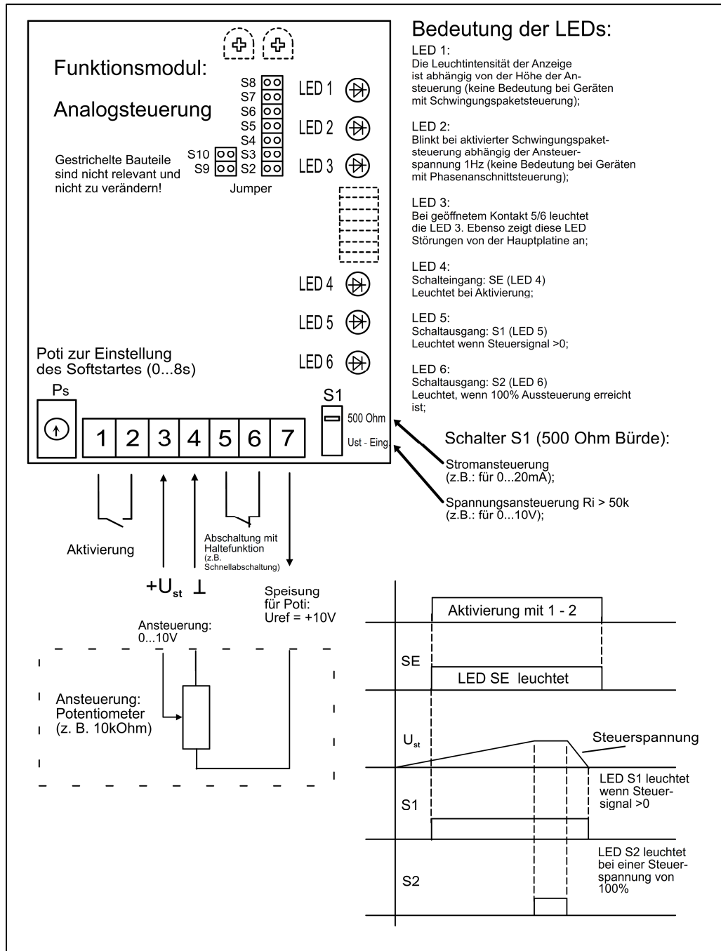
Abbildung 6: Ansteuerung des Funktionsmoduls
