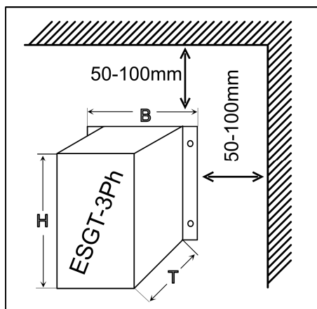
Abbildung 1: Mindestabstand zu anderen Bauteilen am Beispiel ESGT-3Ph
