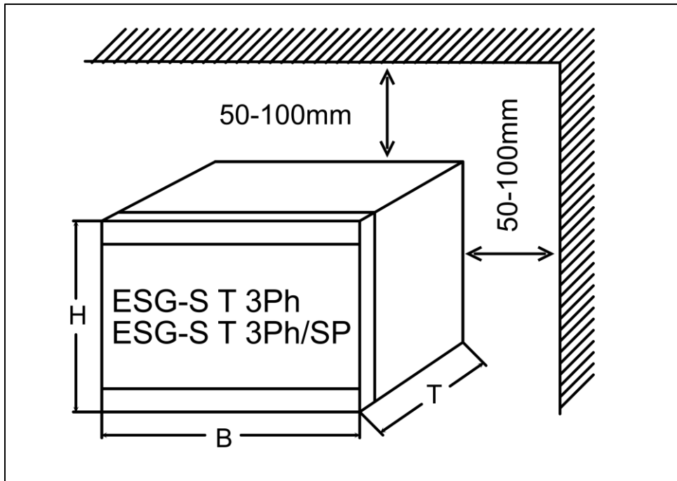
Abbildung 2: Mindestabstand ESG-ST-3ph
