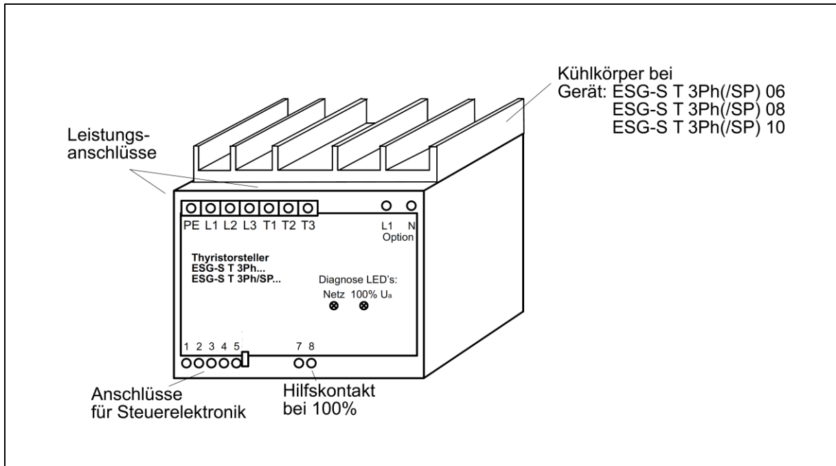
Abbildung 1: Prinzipieller Aufbau des ESG-ST-3ph
