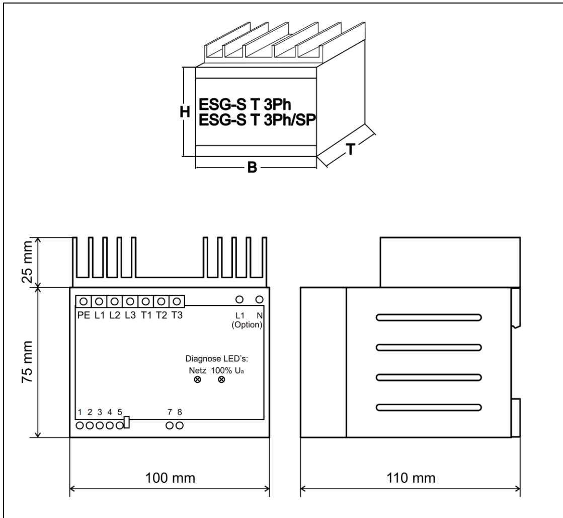
Abbildung 5: Abmessungen des ESG-ST-3ph und ESG-ST-3ph/SP
