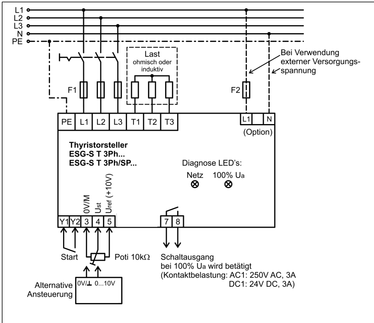
Abbildung 4: Grundschtaltung
