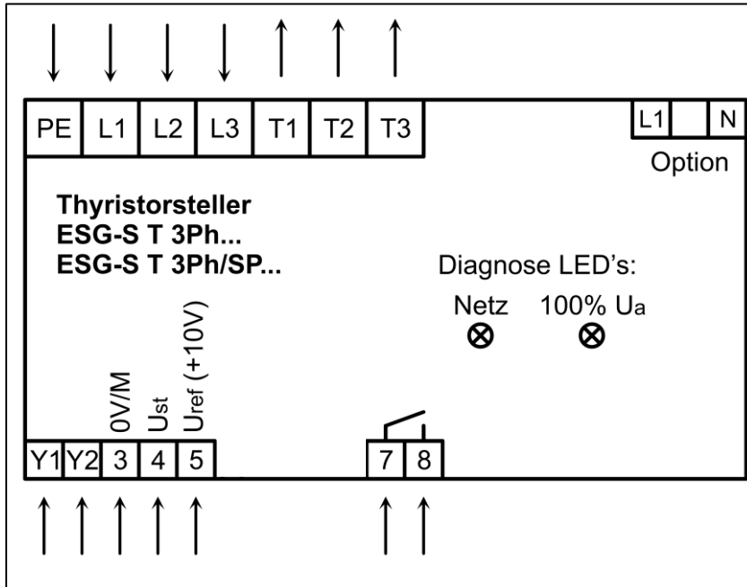
Abbildung 3: Schematische Darstellung der Geräte-Front
