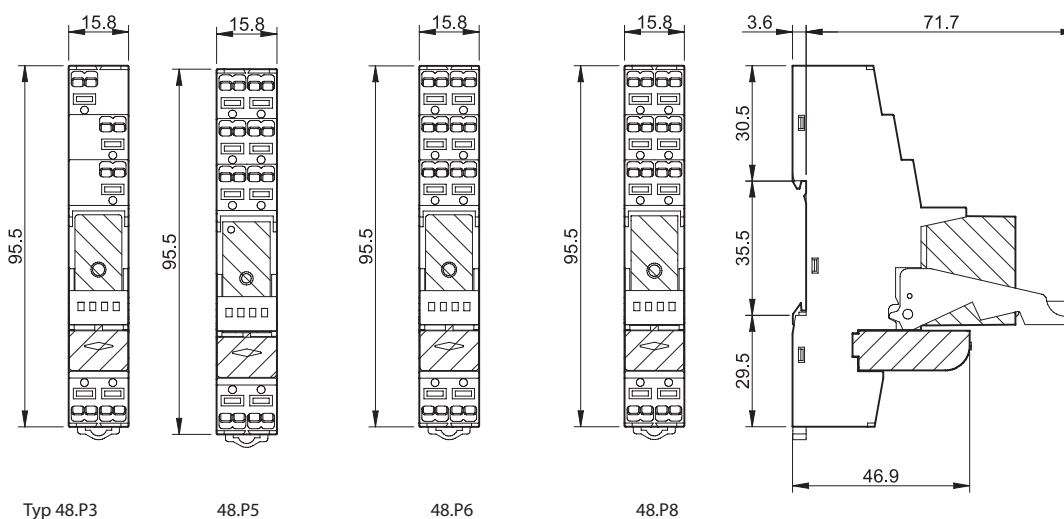
Push-In - Klemmen
